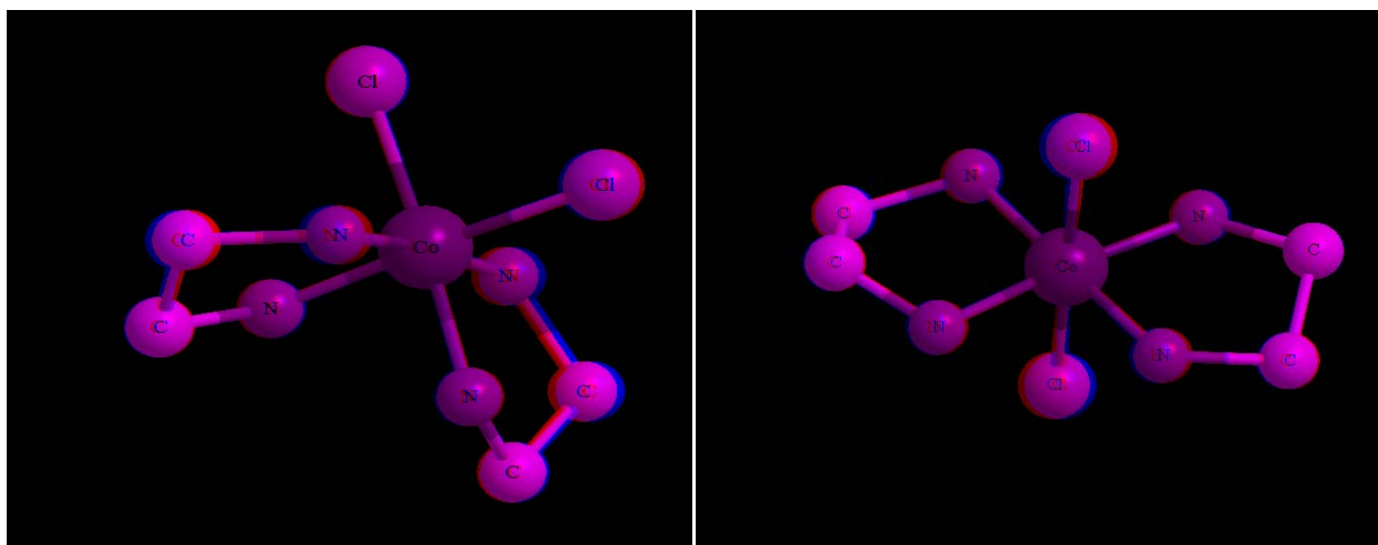
cis-[Co(en) 2 (Cl) 2 ] +
